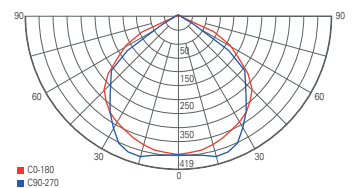
Lichtverteilungskurve
