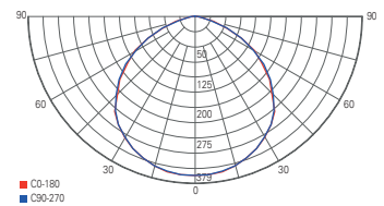
Lichtverteilungskurve 732101
