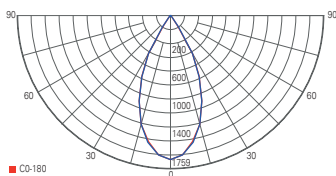
Lichtverteilungskurve
