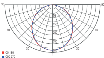
Lichtverteilungskurve LINEAR 60
