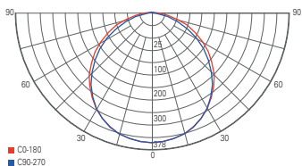
Lichtverteilungskurve 565321, 565368
