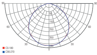
Lichtverteilungskurve 732041
