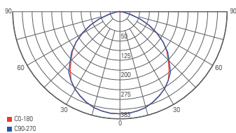
Lichtverteilungskurve 732103
