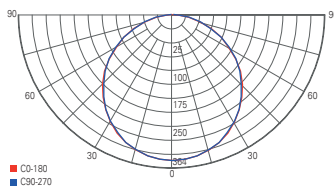
Lichtverteilungskurve LINEAR 100
