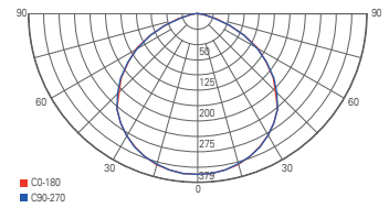
Lichtverteilungskurve 732100
