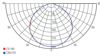
Lichtverteilungskurve 732096
