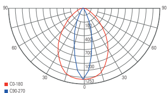
Lichtverteilungskurve 732064
