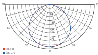
Lichtverteilungskurve 732098
