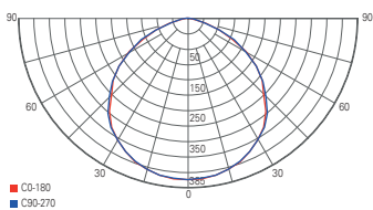
Lichtverteilungskurve 732102
