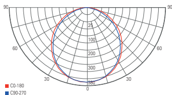
Lichtverteilungskurve 565323, 565370
